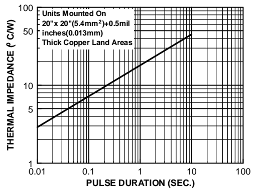
Thermal Impedance
