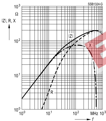
B82483-B1121-A
