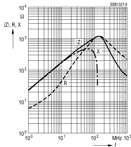
B82483-B1102-A
