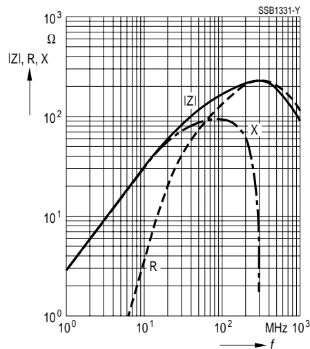
B82485-B1151-A
