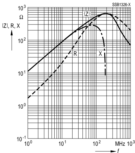
B82483-B1601-A
