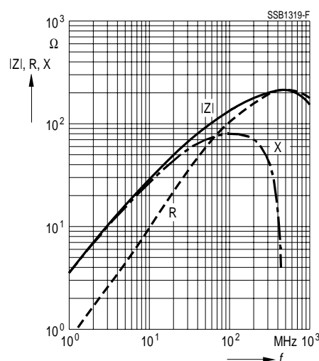
B82482-B1121-A
