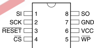
SOIC
