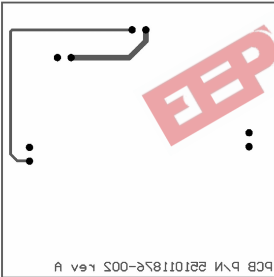
Bottom Layer
