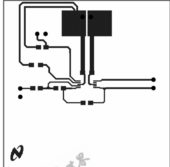
Top Layer
