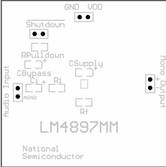
Top Overlay
