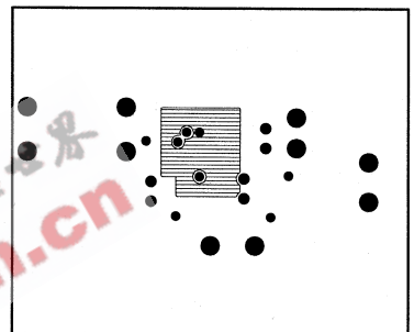
Inner Layer V DD
