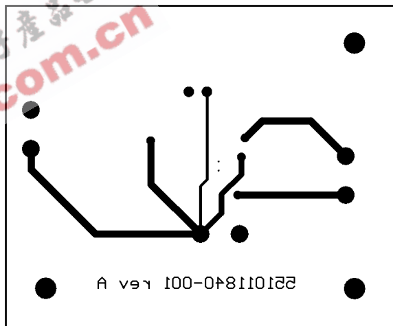
Bottom Layer
