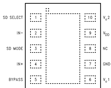
LLP Package
