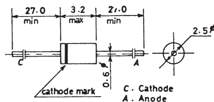
Package Dimensions 1209 (unit : mm)
