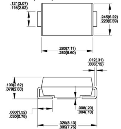
DO-214AB (SMC)
