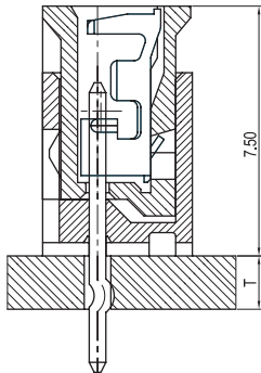
PCB ASS'Y
