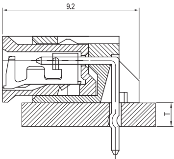
PCB ASS'Y
