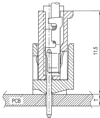
PCB ASS'Y
