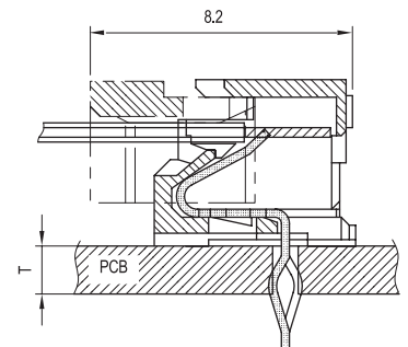
PCB ASS'Y
