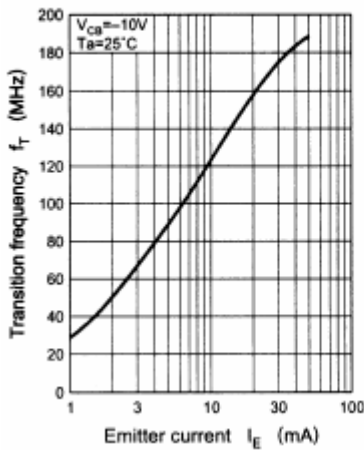
f_T - I_E
