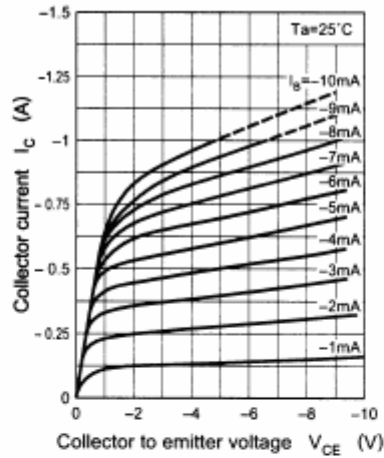
I_C - V_{CE}
