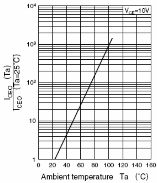
I_{CEO} - T_a
