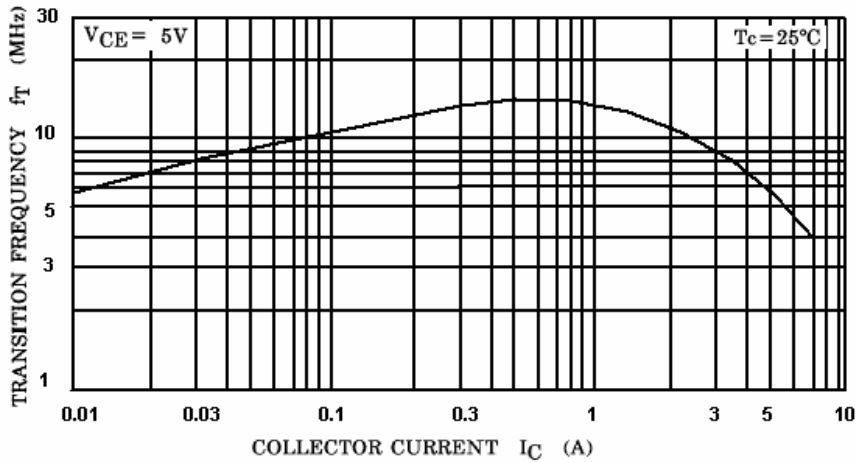
Fig.5 f_T - I_C
