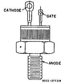
JEDEC TO-208 AA
