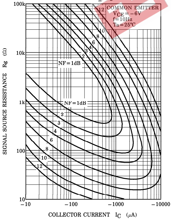
NF - R g , I C
