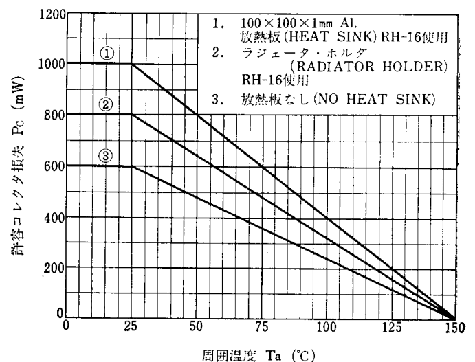
P_C - T_a
