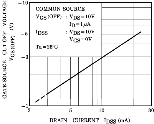
V GS (OFF) - I DSS
