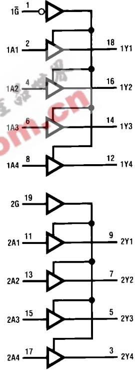
DM74ALS241A
