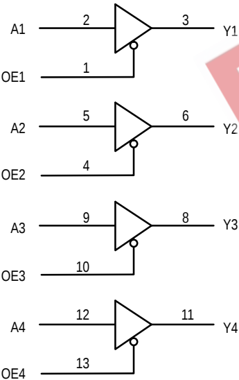
HC125A Active-Low Output Enables
