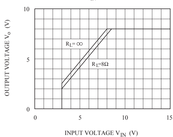
Fig.6-3 V_{IN} - V_o (KIA78R08)
