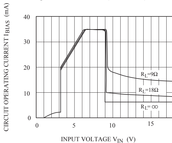
Fig.7-4 V_{IN} - I_{BIAS} (KIA78R09)
