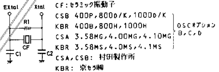
図2-(1) 推奨発振回路(1)/セラミック振動子用
