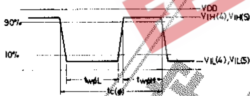
Extal入力時: VIH(5), VIL(4) Xtal入力時: VIH(4), VIL(4) 図1 Extal, Xtal入力波形
