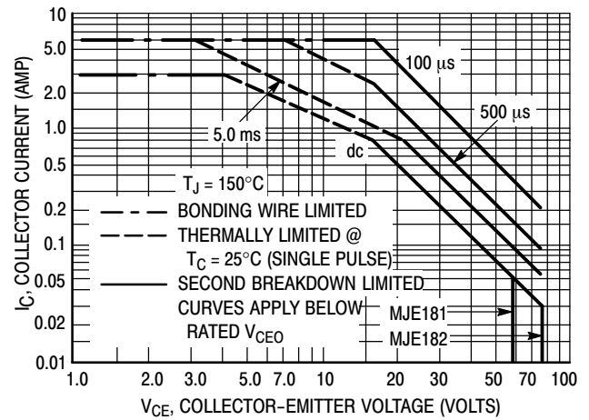
Figure 6. MJE181, MJE182
