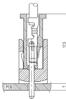
PCB ASS'Y
