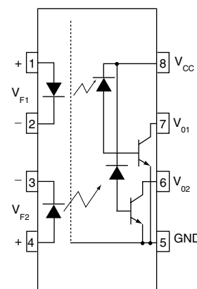
HCPL-2530/HCPL-2531
