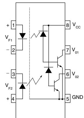
HCPL-2530/HCPL-2531
