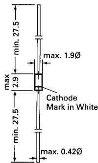
Glass case JEDEC DO-34
