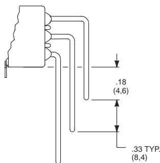
7301MD9ABE Horizontal Actuation 3PDT
