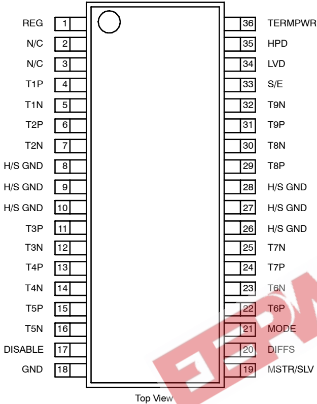
SiP5630 (QSOP-36)
