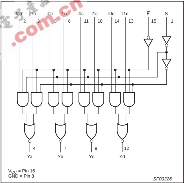
74F158A
