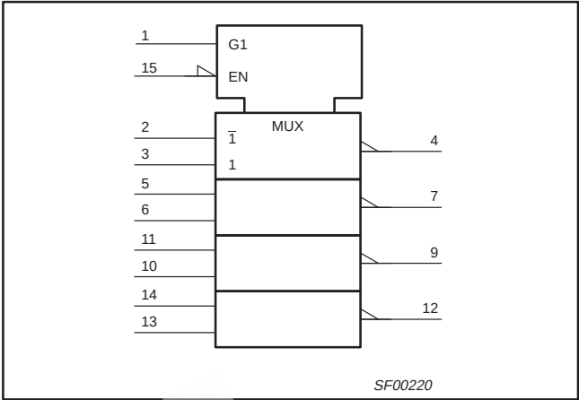
74F158A
