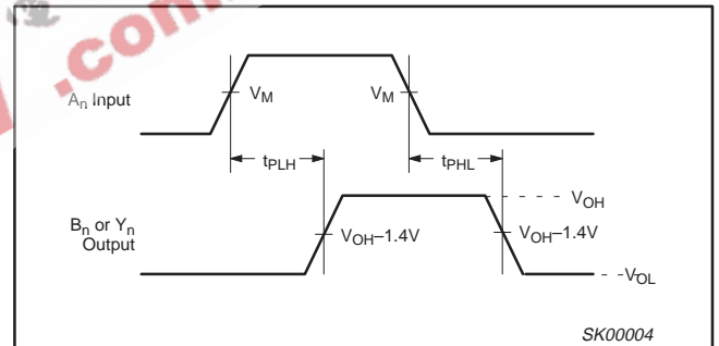
Waveform 2. Propagation Delay for An to Bn or Yn Outputs
