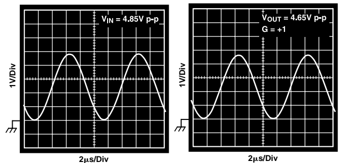
Input V_{IN}
