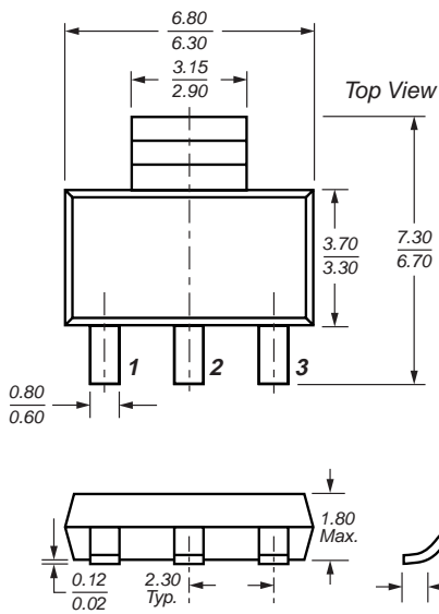
SOT-223
