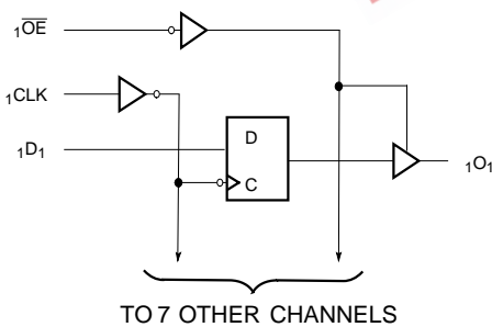
FCT162374-1
