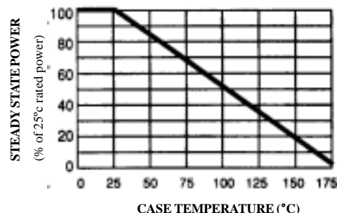
CASE TEMPERATURE (°C)
