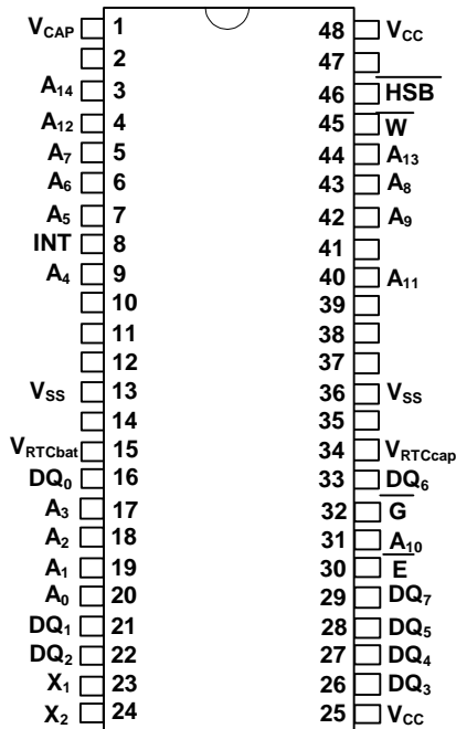
48 Pin SSOP
