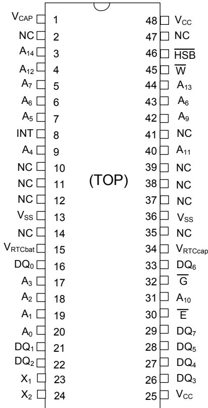
48 Pin SSOP
