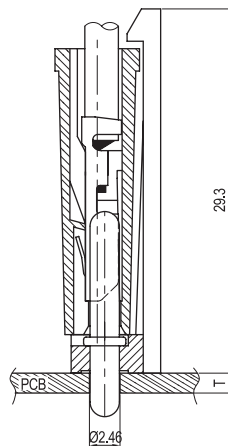
PCB ASS'Y
