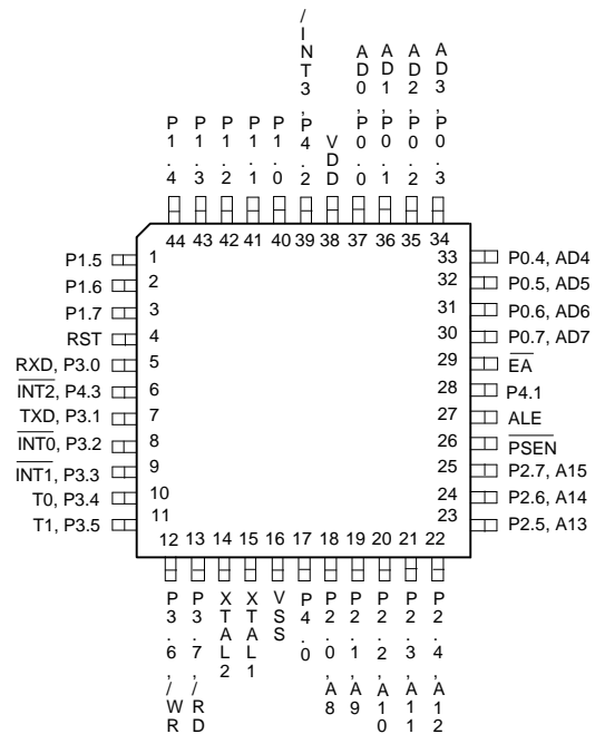
44-Pin QFP (W78C51DF)
