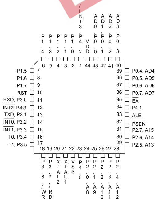
44-Pin PLCC (W78C51DP)
