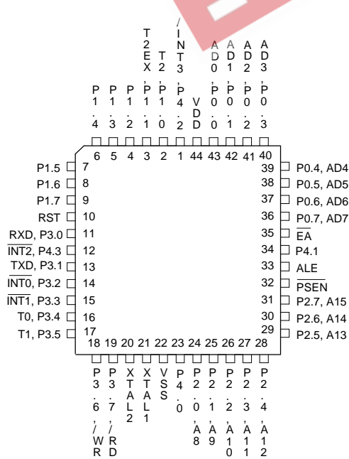
44-Pin PLCC (W78C52DP)
