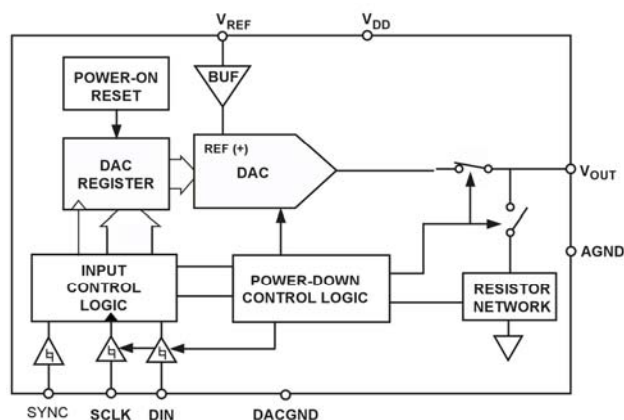
AD5062 8 Ld Sot23.
