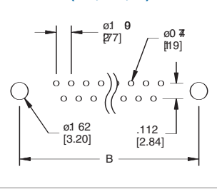
PCB Edge
