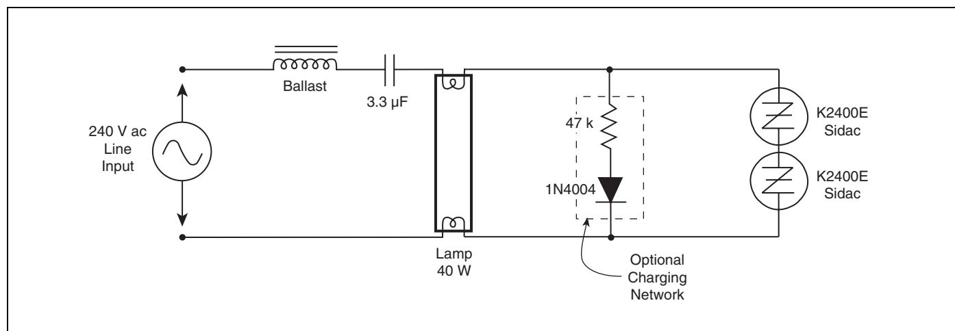
Figure AN1010.5 240 V ac Sidac Circuit
