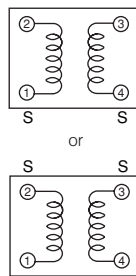
Schematics 結線図
