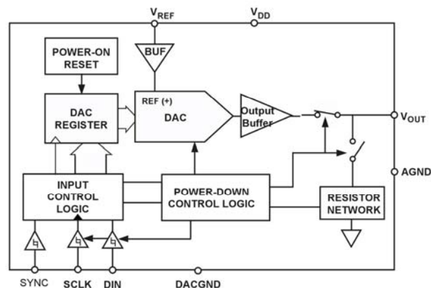
AD5040/AD5060
