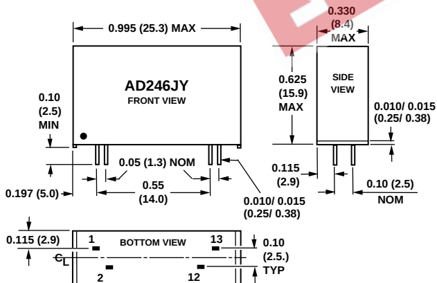
AD246JY Package
