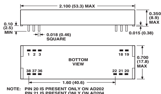
AD202/AD204 DIP Package
