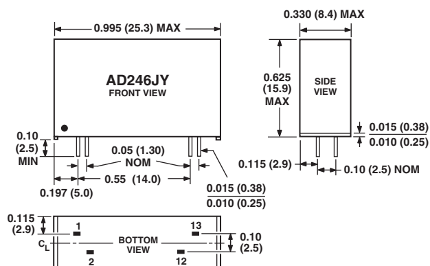
AD246JY Package
