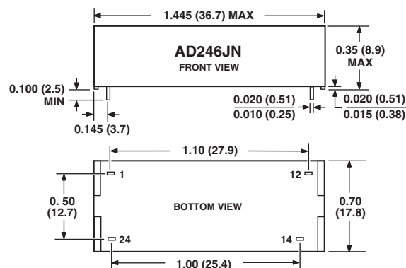
AD246JN Package
