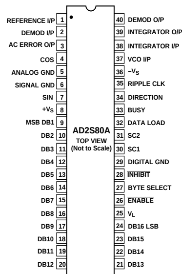
DIP (D) Package
